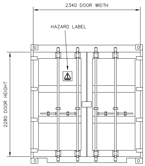
END ELEVATION
