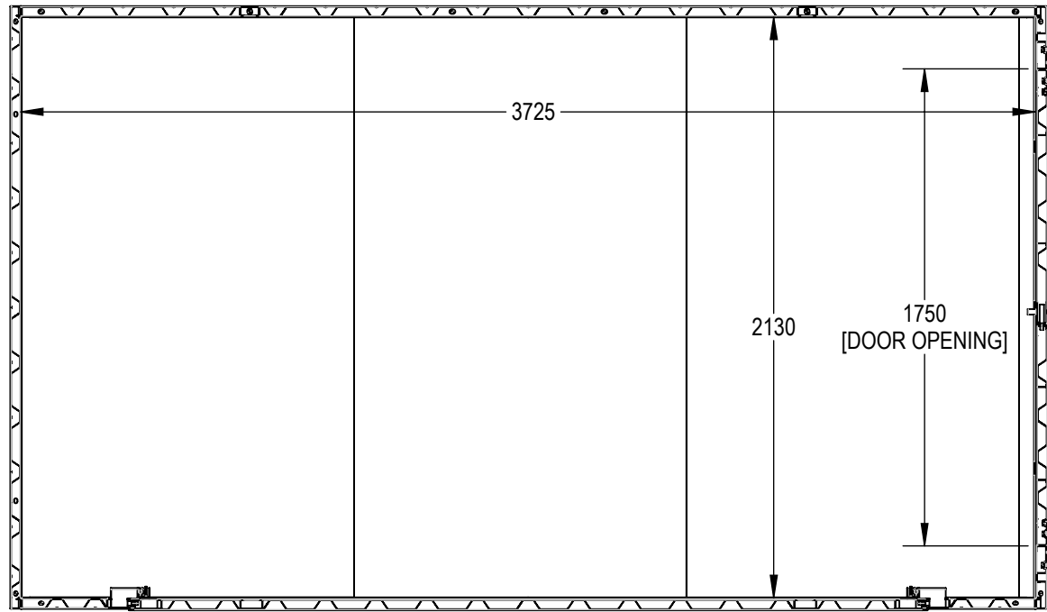
SECTION A-A
