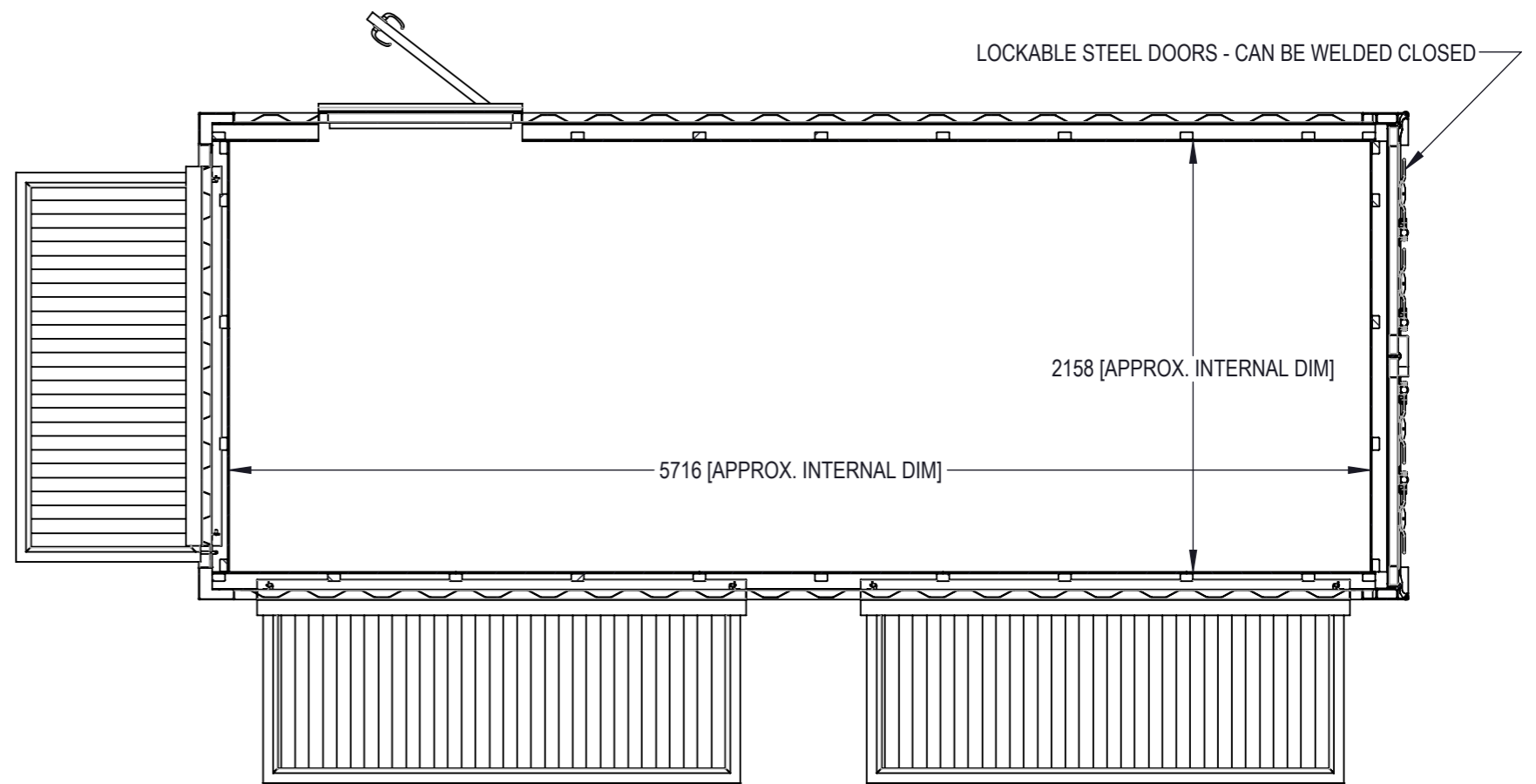
SECTION A-A SCALE 1 : 33
