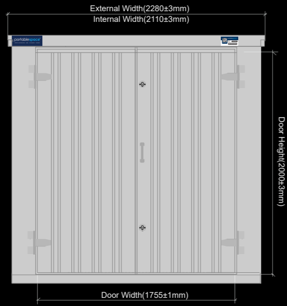
DOOR END
